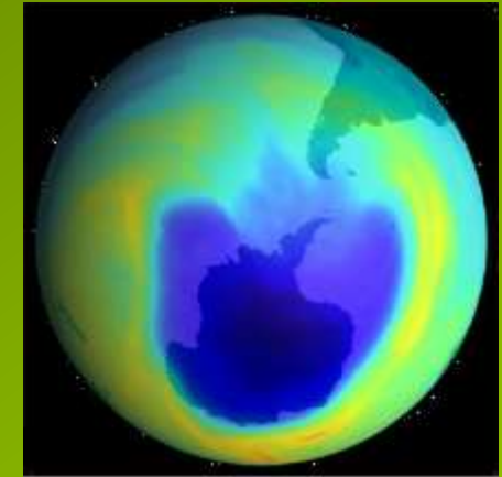
Dziura ozonowa nad biegunem południowym
